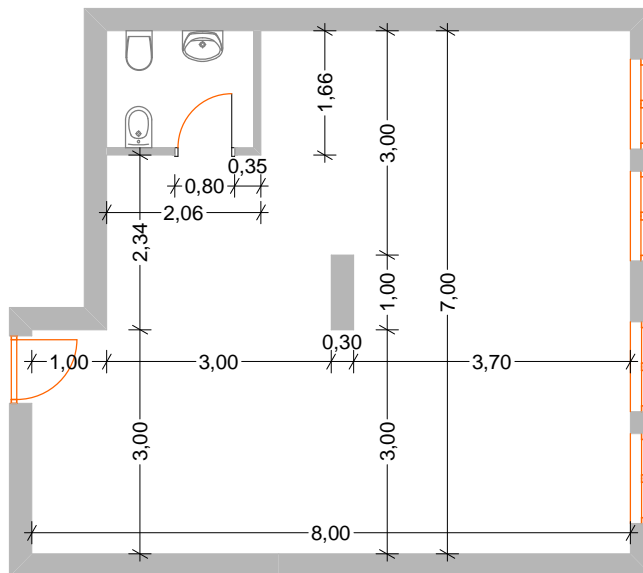
PIANTA STATO DI FATTO
