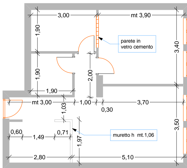
PIANTA DIVISIONE - QUOTATA
